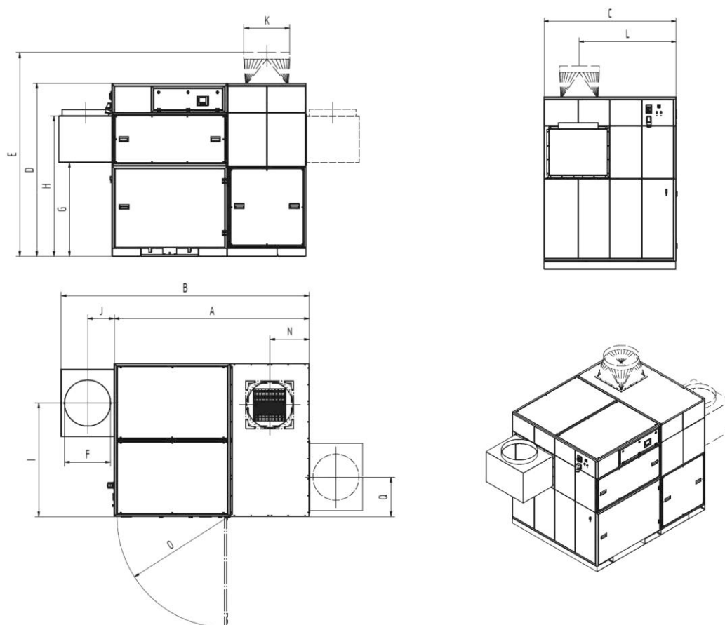
Fig. 56: Disegno quotato 998701370 (998800414, 998800463)
