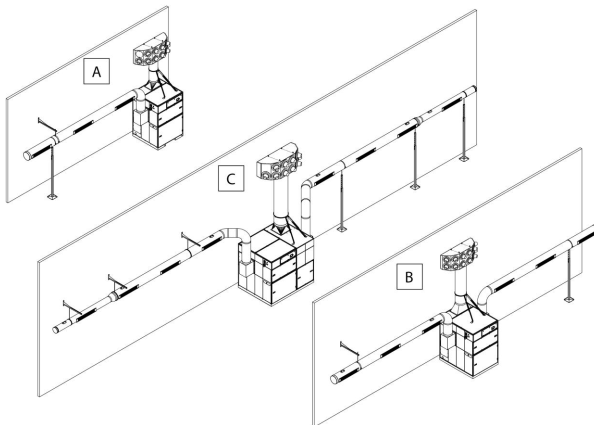
Fig. 11: Montaggio – Panoramica delle varianti del prodotto
