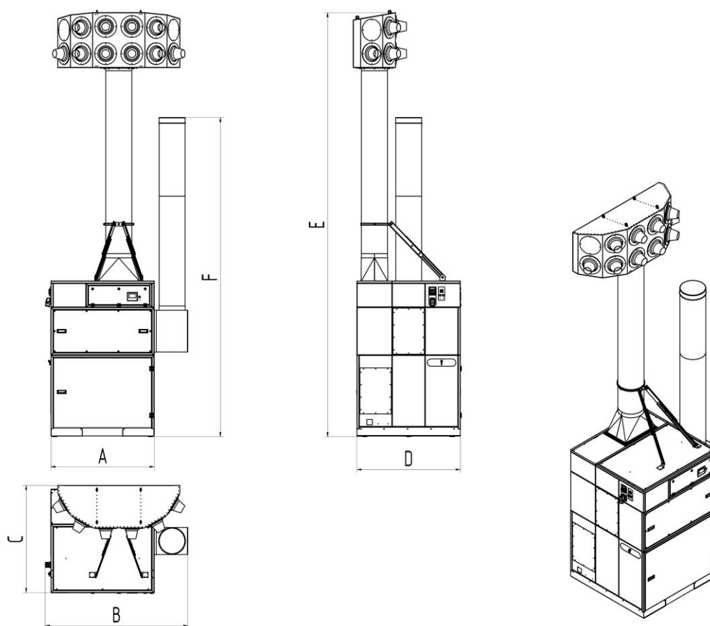
Fig. 60: Disegno quotato – 998800461
