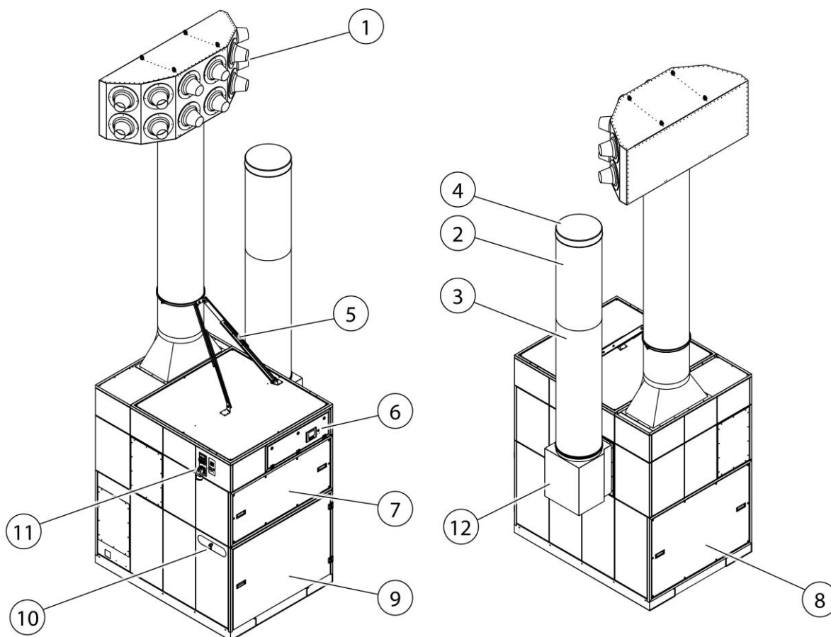
Fig. 5: Descrizione del funzionamento - 998800462
