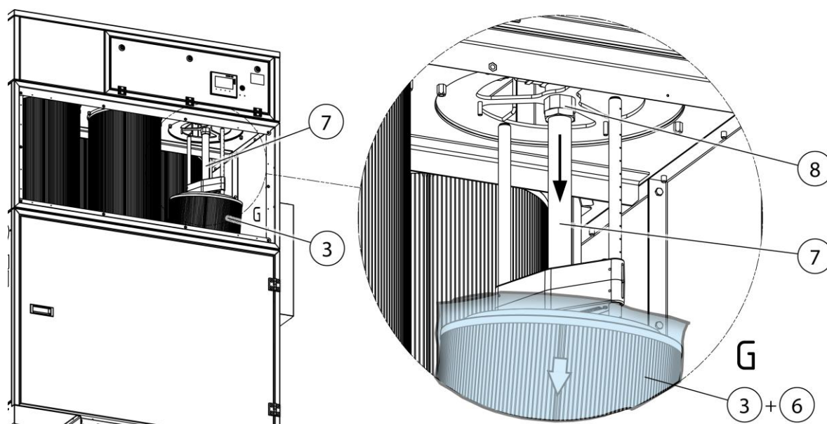
Fig. 41: Smontaggio ugello rotante
