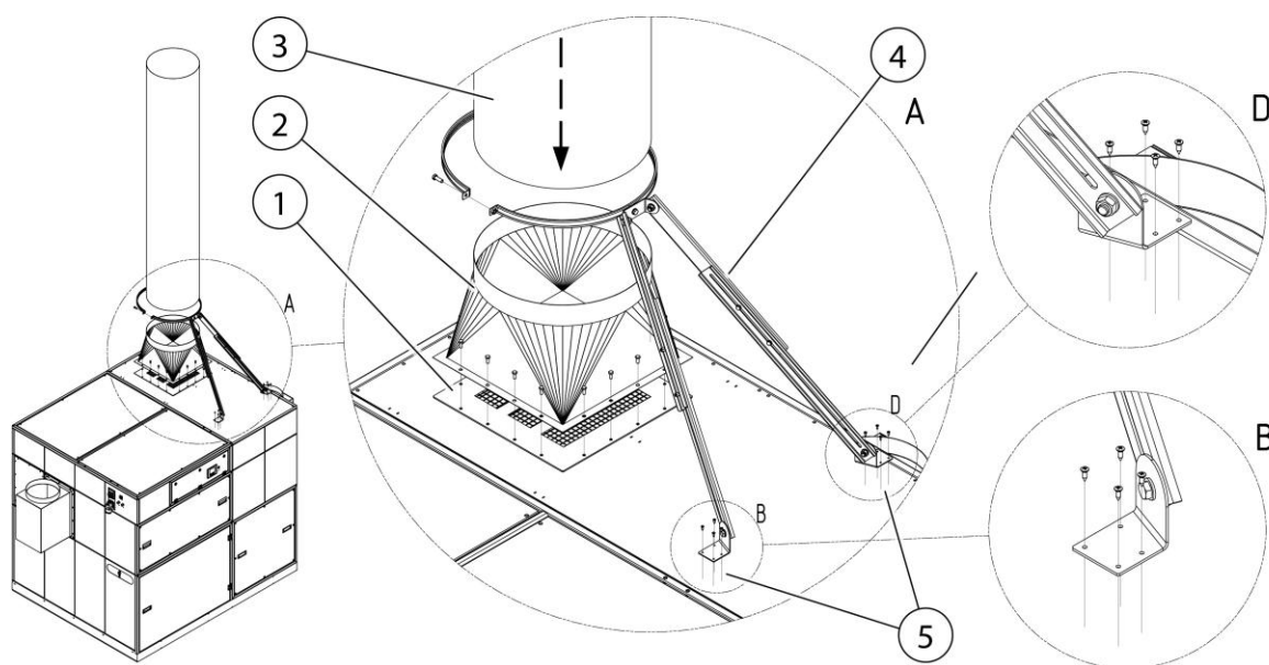
Fig. 12: Montaggio - Unità di scarico
