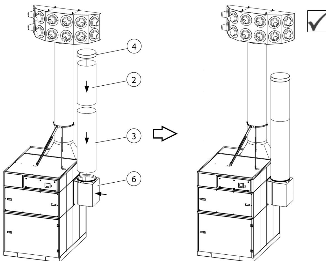
Fig. 17: Posizioni sul prodotto
