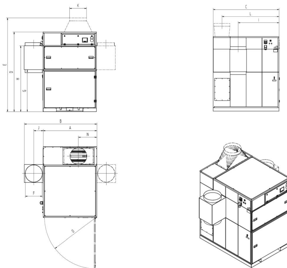
Fig. 55: Disegno quotato 998701371 (998800401, 998800462)
