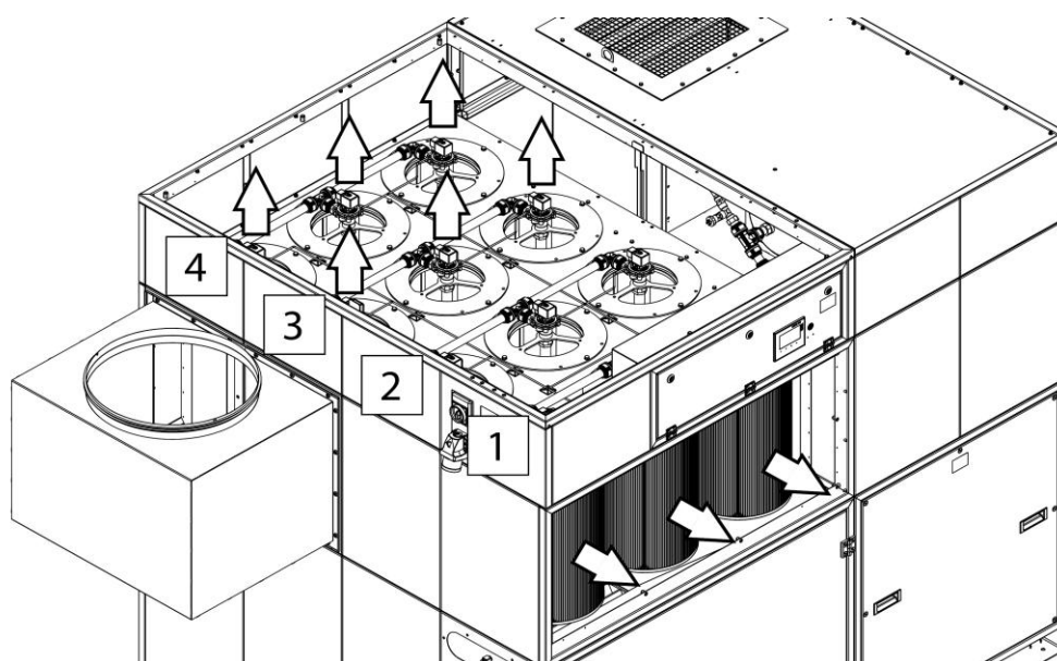
Fig. 39: Cambio filtro
