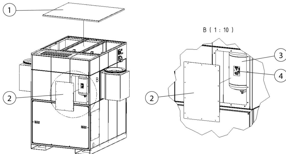
Fig. 52: Accesso al serbatoio dell'aria compressa
