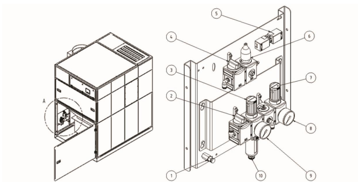
Fig. 10: Unità pneumatica
