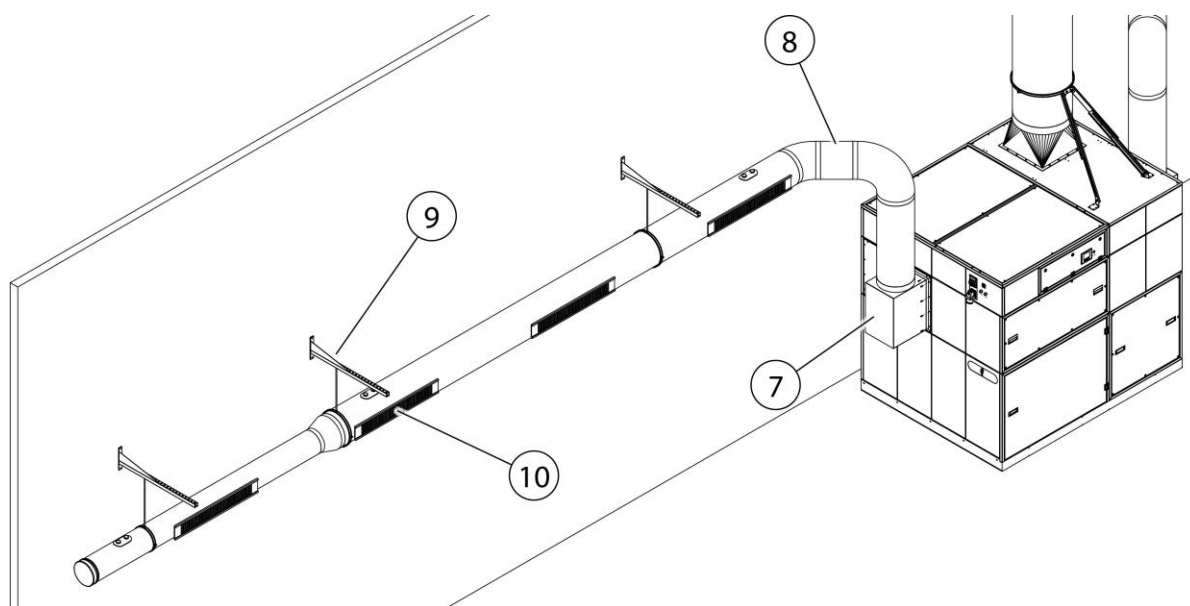
Fig. 14: Montaggio a parete - Tubazione di aspirazione
