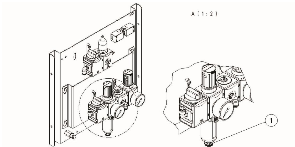
Fig. 49: Valvola di scarico della condensa unità di manutenzione pneumatica
