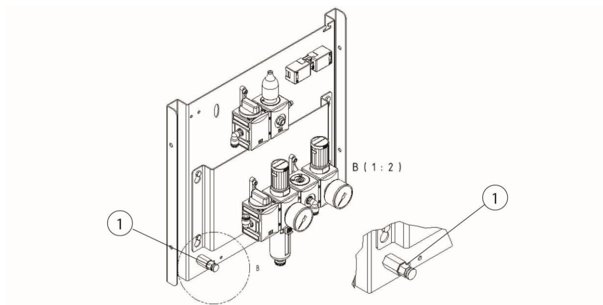
Fig. 48: Valvola di scarico condensa serbatoio dell'aria compressa
