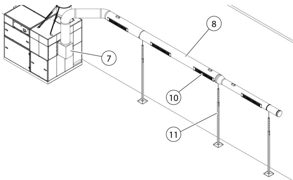
Fig. 15: Montaggio sul pavimento - Tubazione di aspirazione
