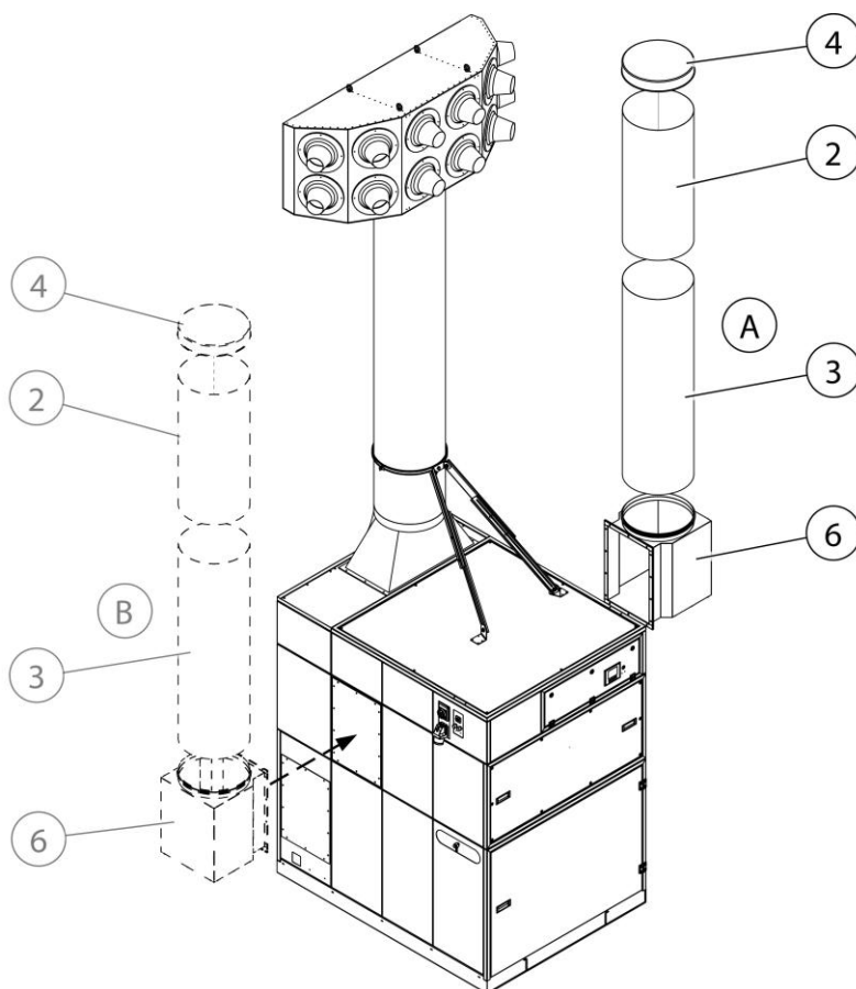
Fig. 16: Montaggio - Collettore di aspirazione
