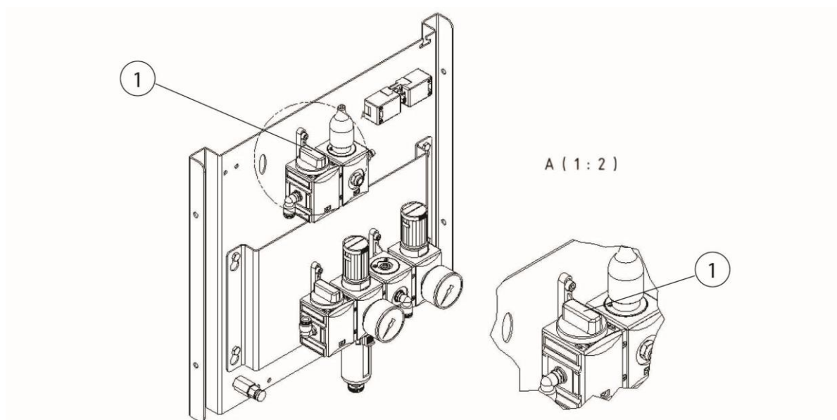
Fig. 34: Valvola pneumatica collettore di polvere
