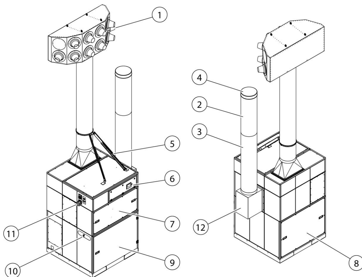
Fig. 4: Descrizione del funzionamento - 998800461
